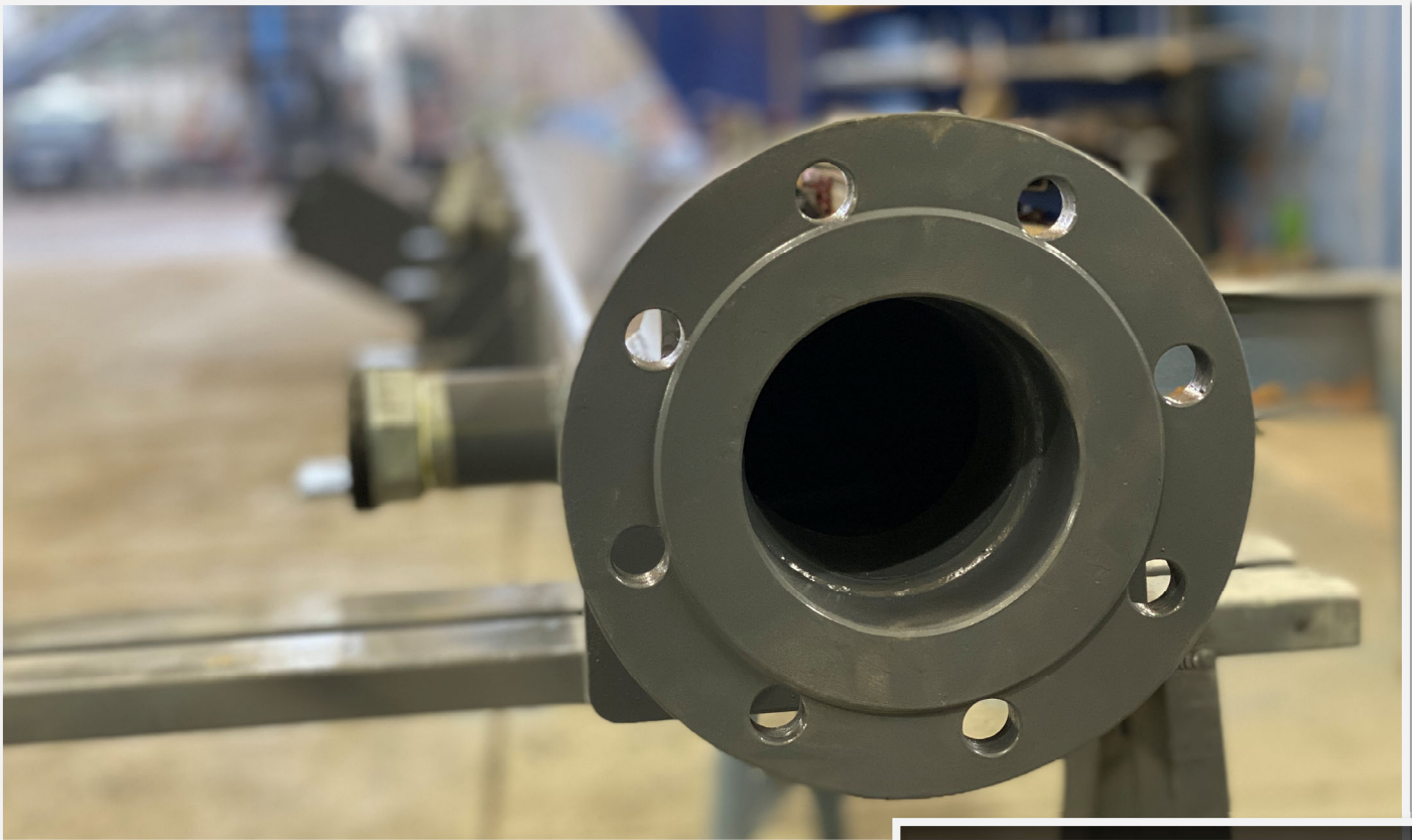
WASCHWASSERZUFUHR DN100/PN10
