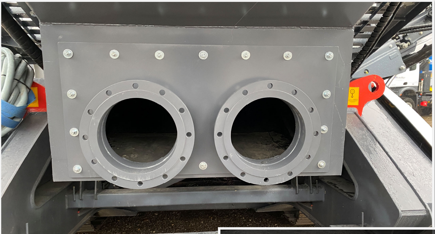
ABGANG SAND-WASSERGEMISCH 2X DN300/PN10
