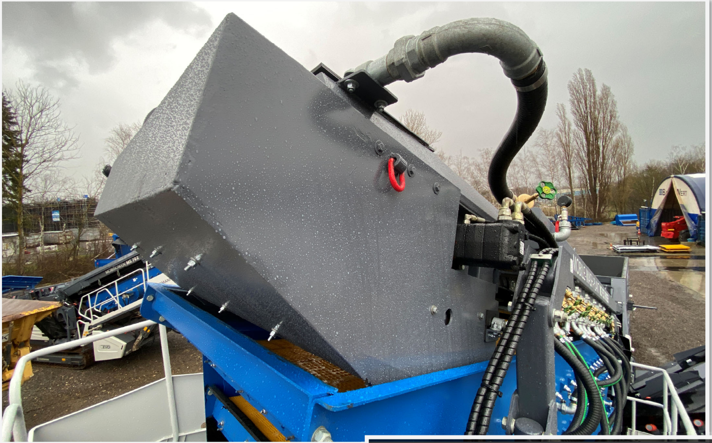
AUFLÖSESCHURRE MIT 2" WASSERZUFUHR
